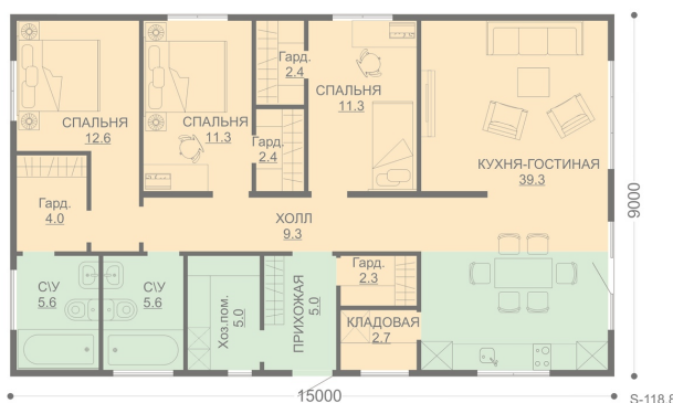
ПЛАН 1-ГО ЭТАЖА
