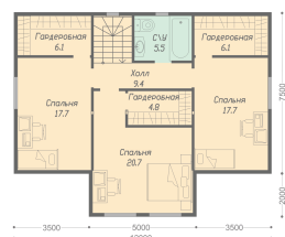
План второго этажа
