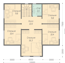
План второго этажа
