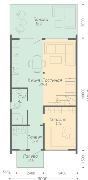
ПЛАН ПЕРВОГО ЭТАЖА
