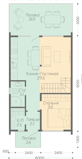
ПЛАН ПЕРВОГО ЭТАЖА
