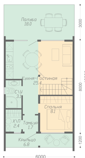
ПЛАН ПЕРВОГО ЭТАЖА
