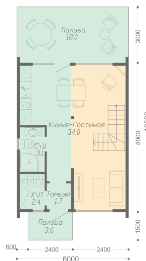
ПЛАН ПЕРВОГО ЭТАЖА
