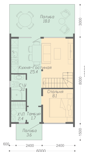
ПЛАН ПЕРВОГО ЭТАЖА
