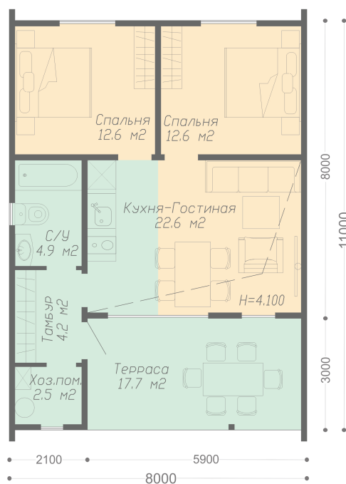
ПЛАН 1-ГО ЭТАЖА
